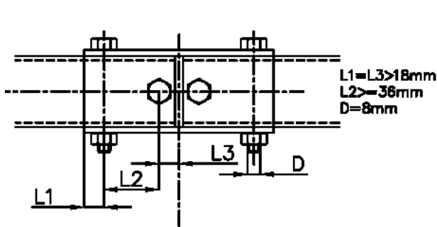
Dessin/Drawing 253-41
